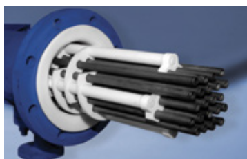
Теплообменники из карбида кремния, максимальная теплопроводность несмотря на компактную конструкцию
